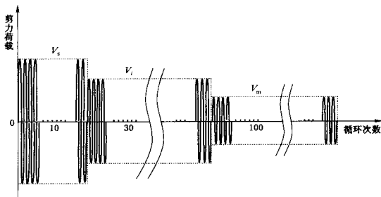
图 F.2 低周反复剪力荷载试验波形
