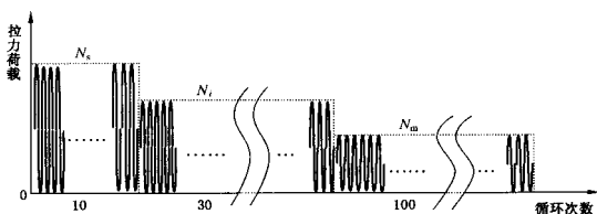
图 F.1 低周反复拉力荷载试验波形
