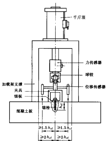
图 E.1 抗拉试验加载设备示意图
