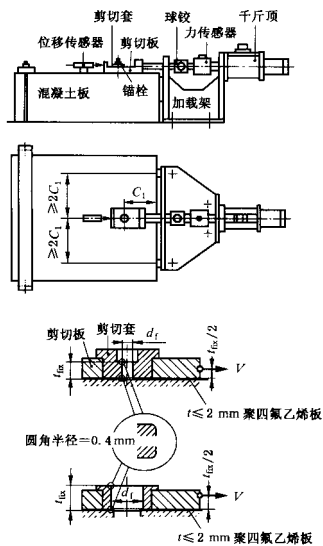
图 E.2 剪切试验加载设备示意图
