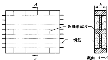
图 B.1 开裂混凝土试件配筋及裂缝形成片
